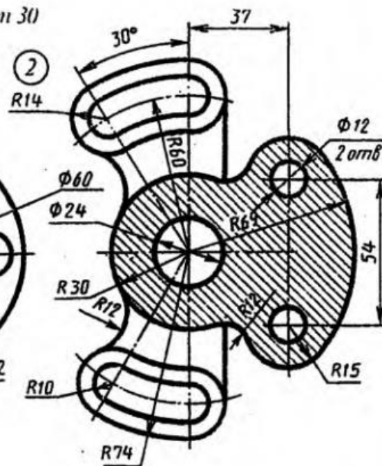
Корпус
