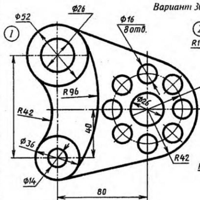
Пластина
